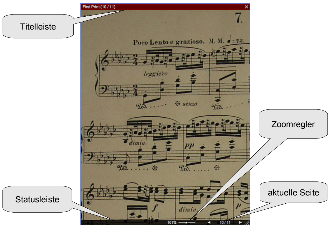
Abbildung 4: Quellenfenster
