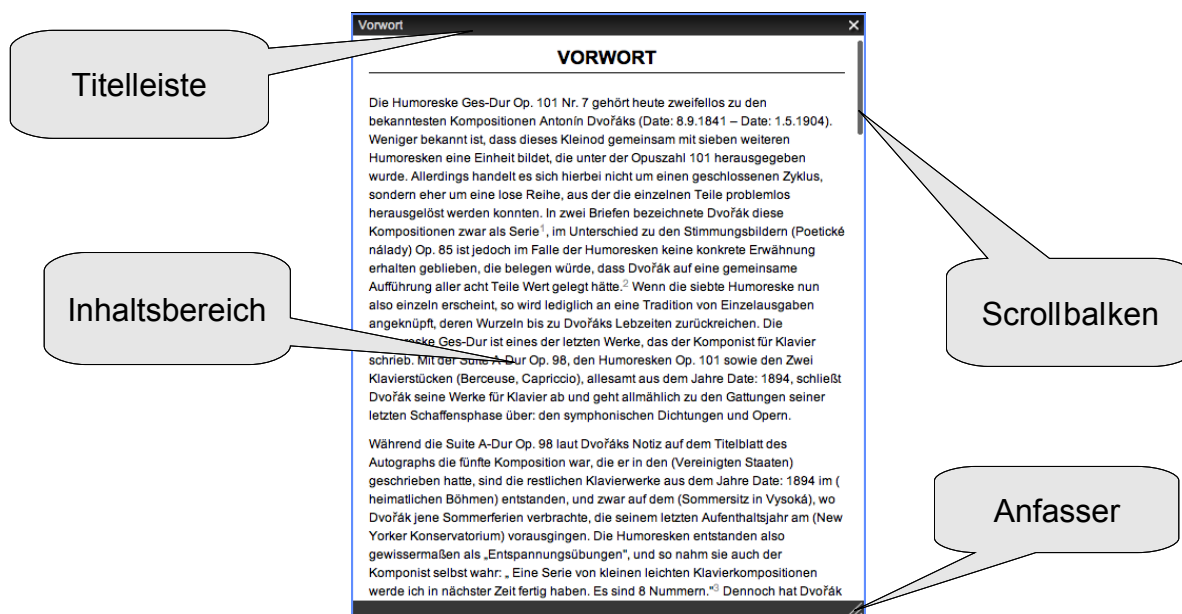
Abbildung 3: Textfenster
